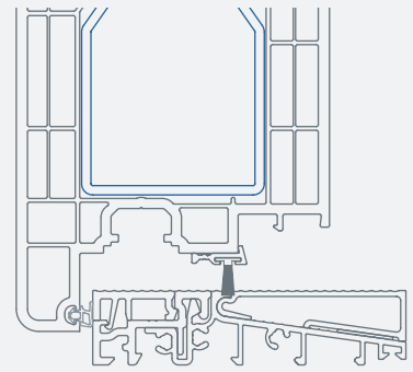
Variante ouvrant vers l'extérieur
